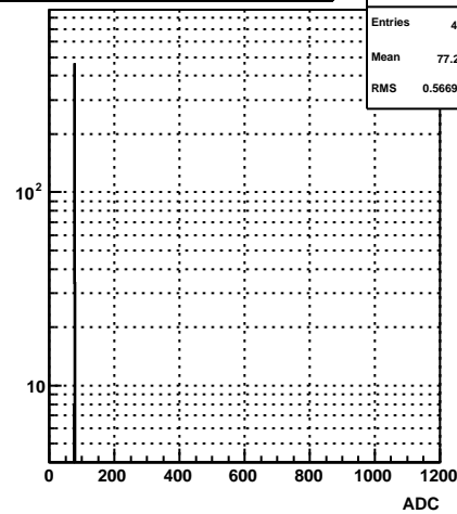
ZDC SMD West Vert ADC, strip 8
